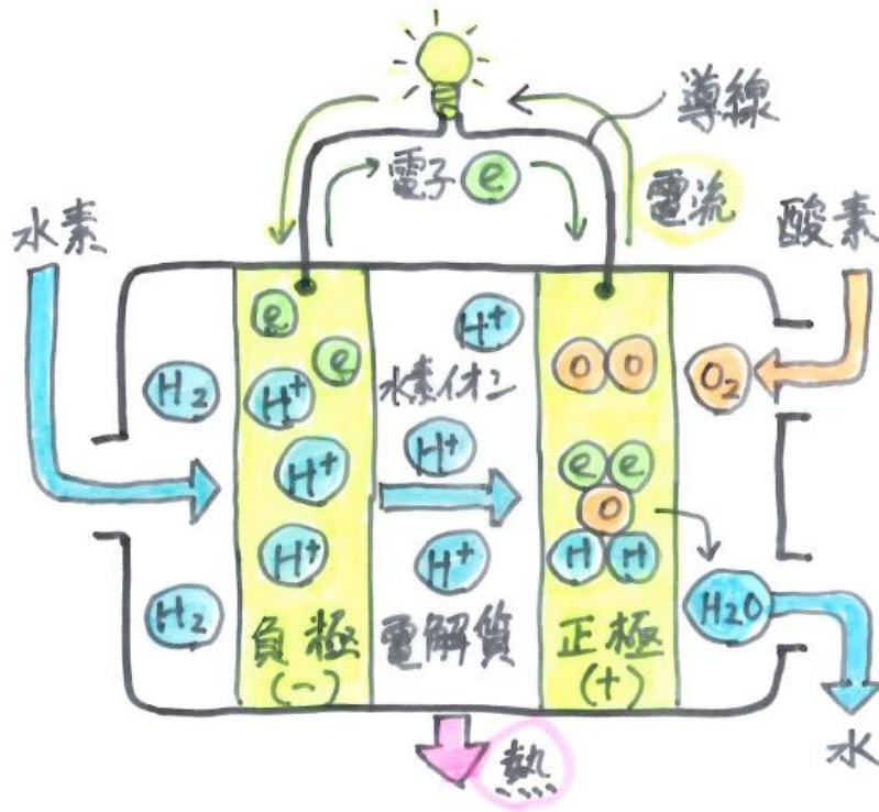
図 燃料電池の構造
