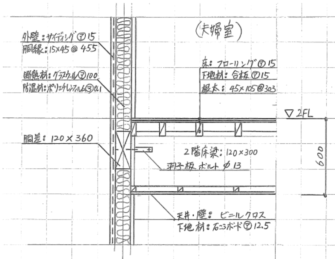
図2 2階梁部の部分詳細図
