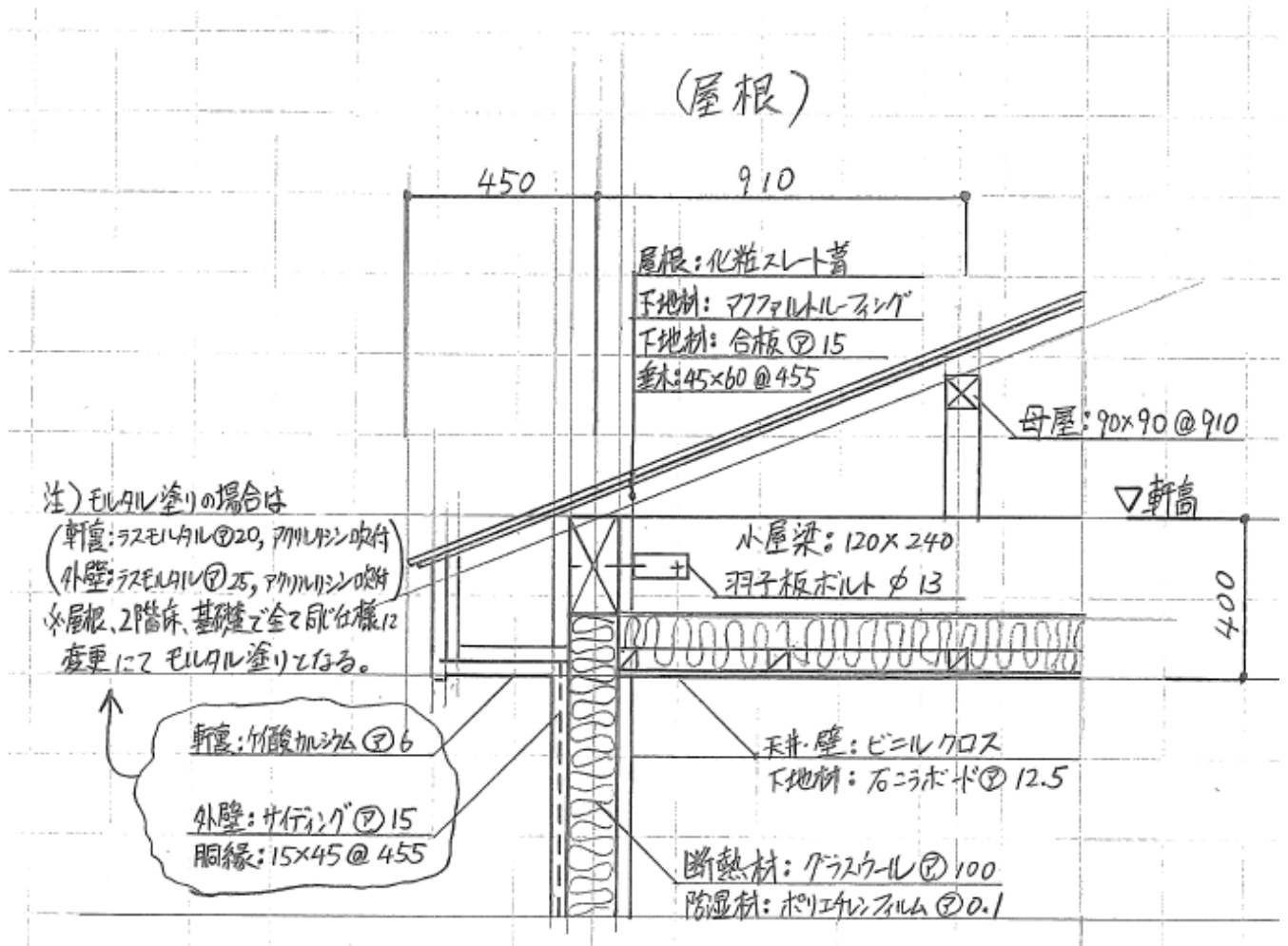
図3 屋根梁部の部分詳細図
