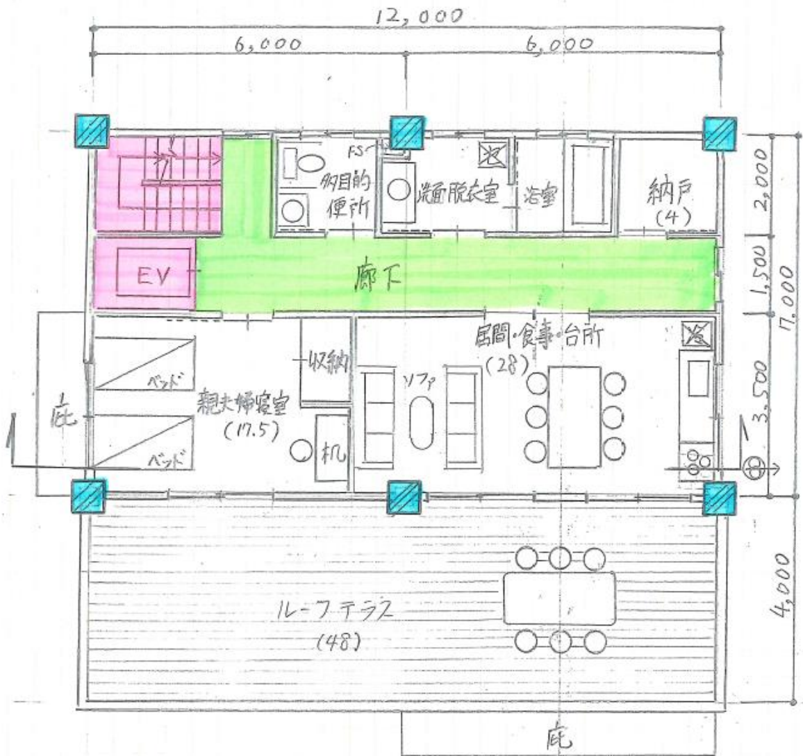
図2 2階平面図の解答
