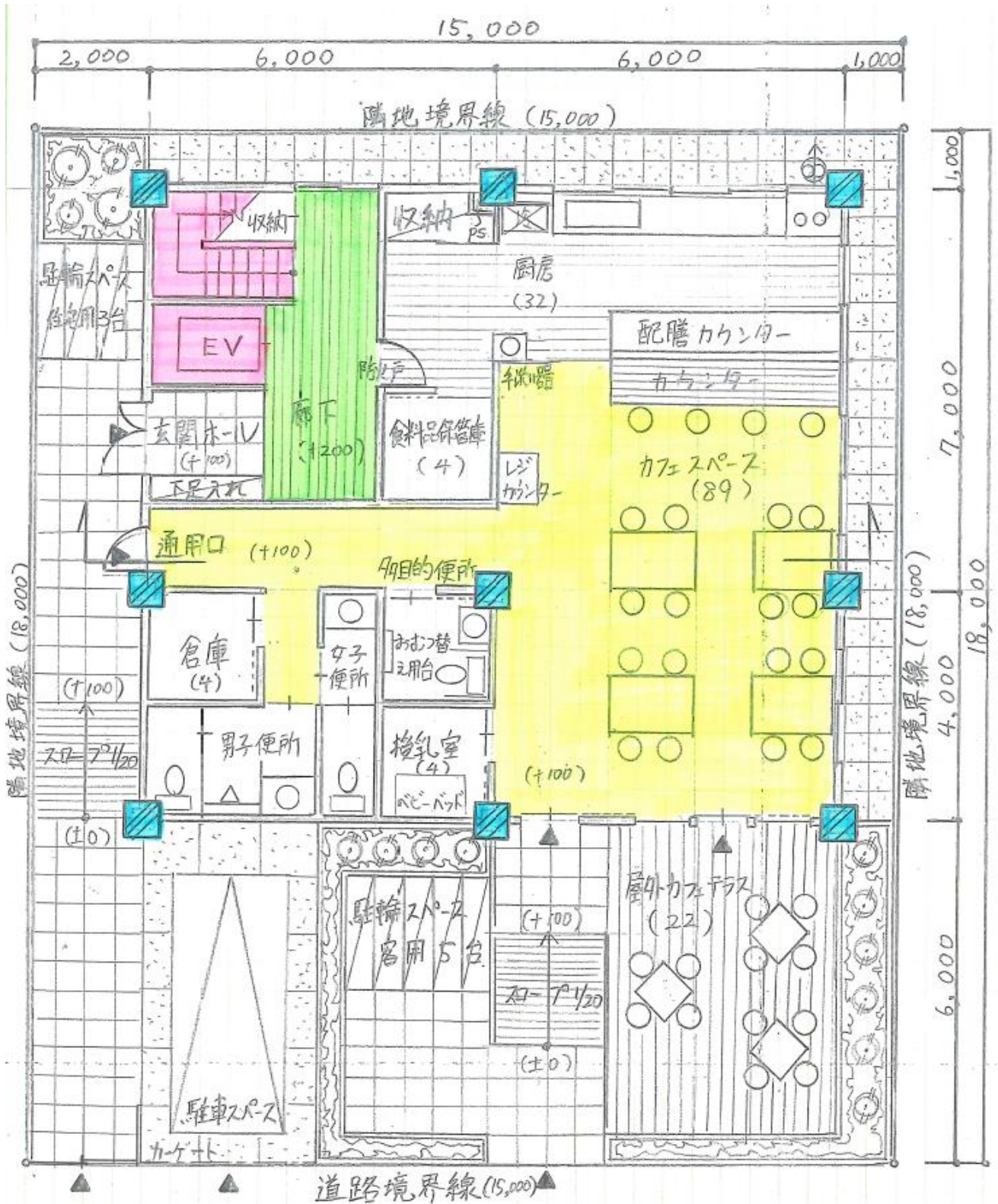
図1 1階平面図兼配置図の解答
