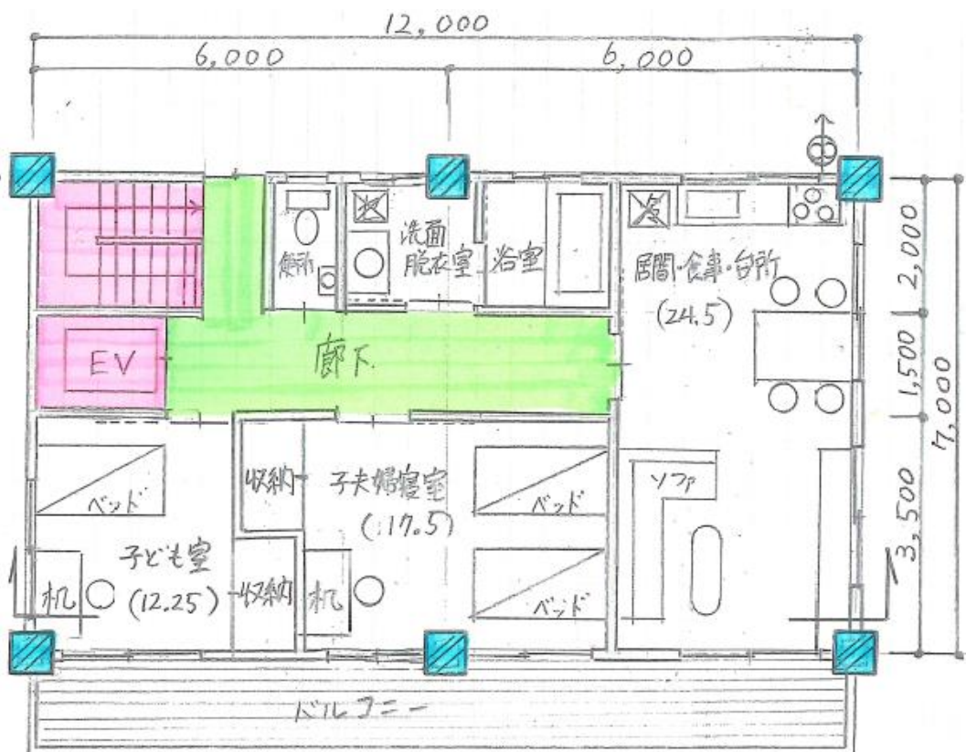
図3 3階平面図の解答
