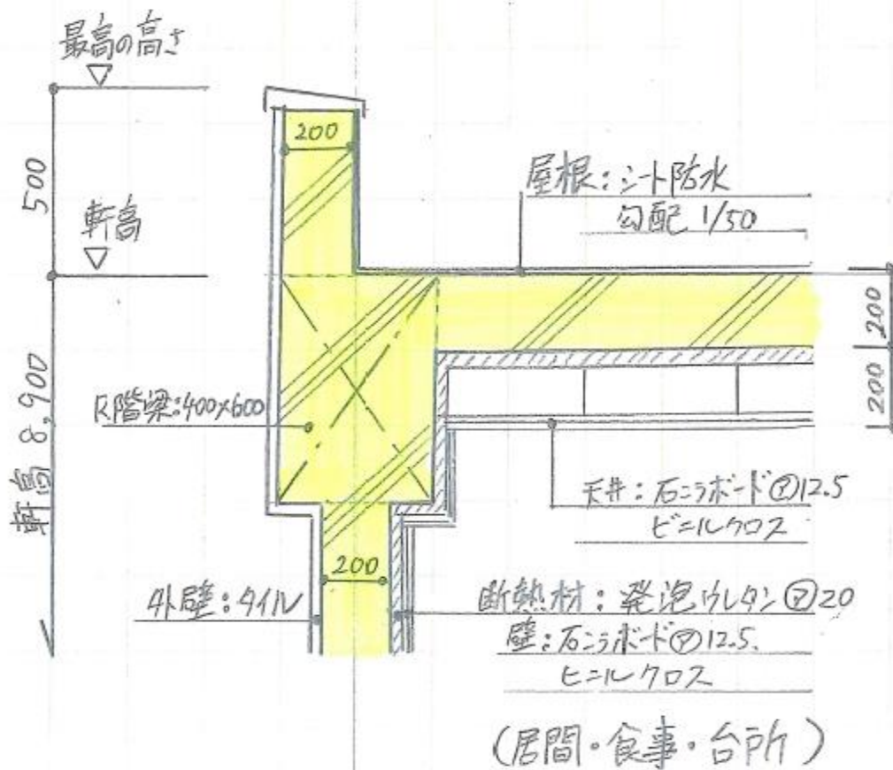
図3 R梁部の部分詳細図
