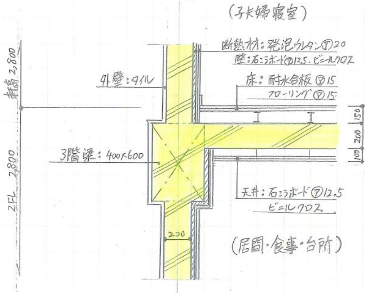
図2 3階梁部の部分詳細図
