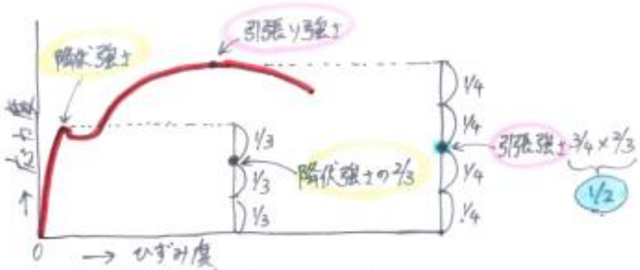
図 鋼材の許容応力
