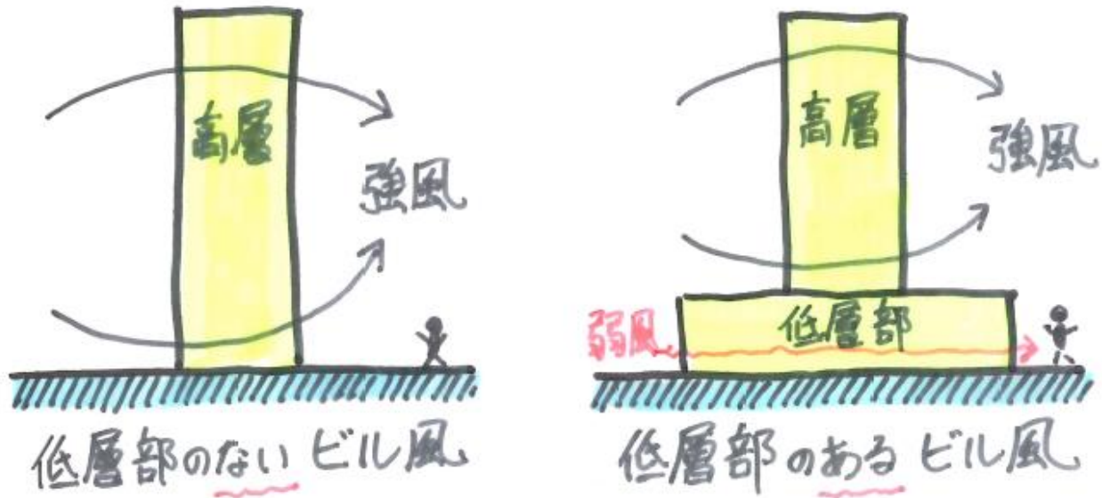
図 低層部の有無による高層建物のビル風
