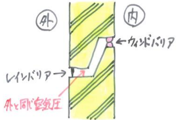
オープンジョイント
