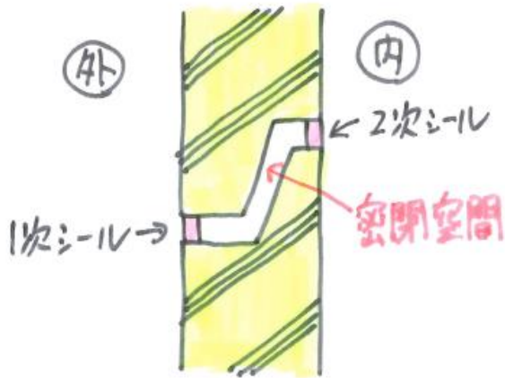
フィルドジョイント
